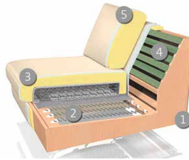
Das Design des hier abgebildeten Querschnitts entspricht nicht dem Modell dieses Katalogblattes.
